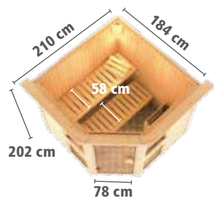
Zeichnung und Maße mit Dachkranz
