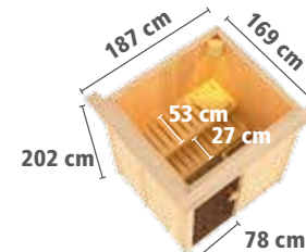
Zeichnung und Maße mit Dachkranz
