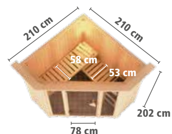
Zeichnung und Maße mit Dachkranz
