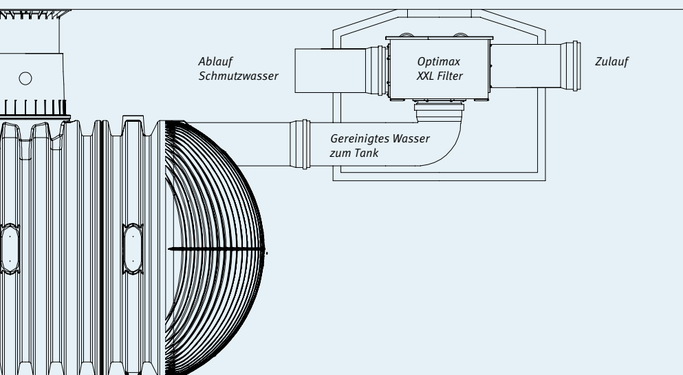
Funktion Filter-Reinigungseinheit
