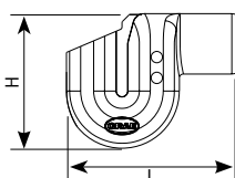
DN 150 1)
