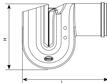
DN 200 / DN 300 2)
