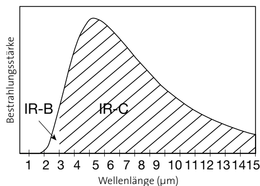
Strahlenspektrum für einen Keramikstrahler
