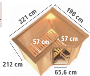
Zeichnung und Maße mit Dachkranz
