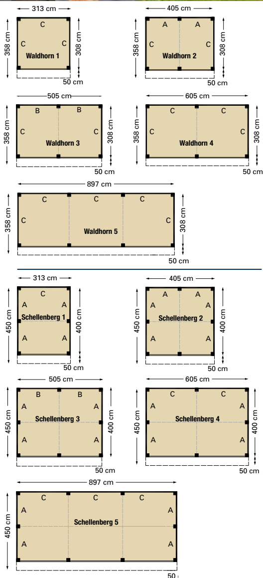
Lieferung Standardausführung ohne Wände und ohne Boden Dacheindeckung: EPDM Folie
