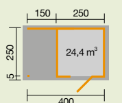
Designhaus „wekaLine“ 413 B
