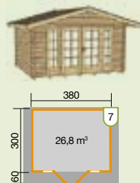
weka Weekendhaus 137 Vordach 60 cm
