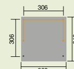
weka Gartenlaube 657 · 657.3535.00.10 · Abb. mit kostenpflichtigem Zubehör (Zusatzfenster, Rück- und Seitenwände)
