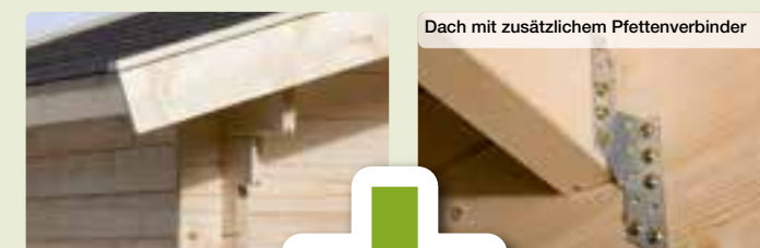
Dach mit zusätzlichem Pfettenverbinder
