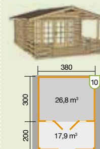
weka Weekendhaus 137 B Vordach 200 cm + Terrasse 200 cm inkl. Stützen, Abschlussblende und Querstrebe
