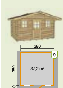
weka Weekendhaus 138 Vordach 60 cm
