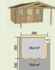
weka Weekendhaus 138 A Vordach 200 cm inkl. Stützen, Abschlussblende und Querstrebe
