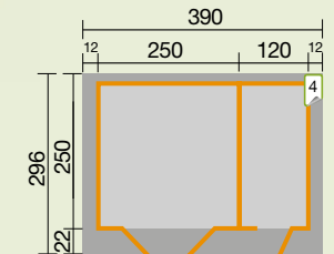
weka Garten- haus 254
