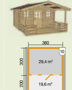
weka Weekendhaus 138 B Vordach 200 cm + Terrasse 200 cm inkl. Stützen, Abschlussblende und Querstrebe
