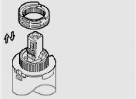
Einstellung der maximalen Temperatur
