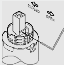
Einstellung der Durchflussmenge
