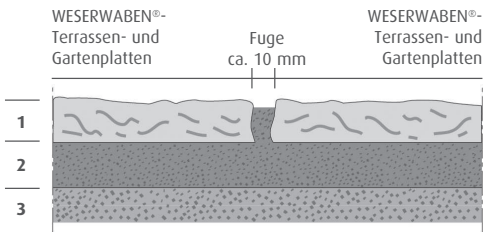
Abb. 1: Prinzip-Skizze Terrassenplatten Opus und Solum
