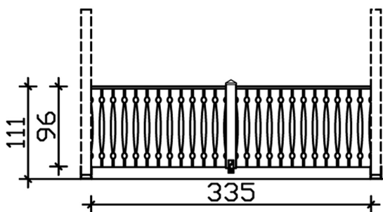
Bemassung
