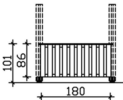
Bemassung
